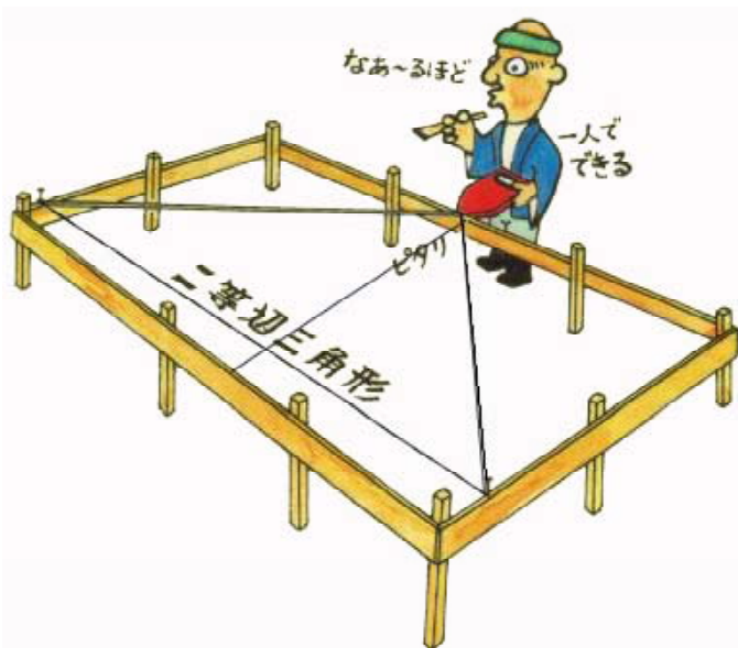
おおがね巻尺
